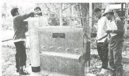
ติดตั้งเครื่องกรองน้ำพร้อมถังบำบัดน้ำ
